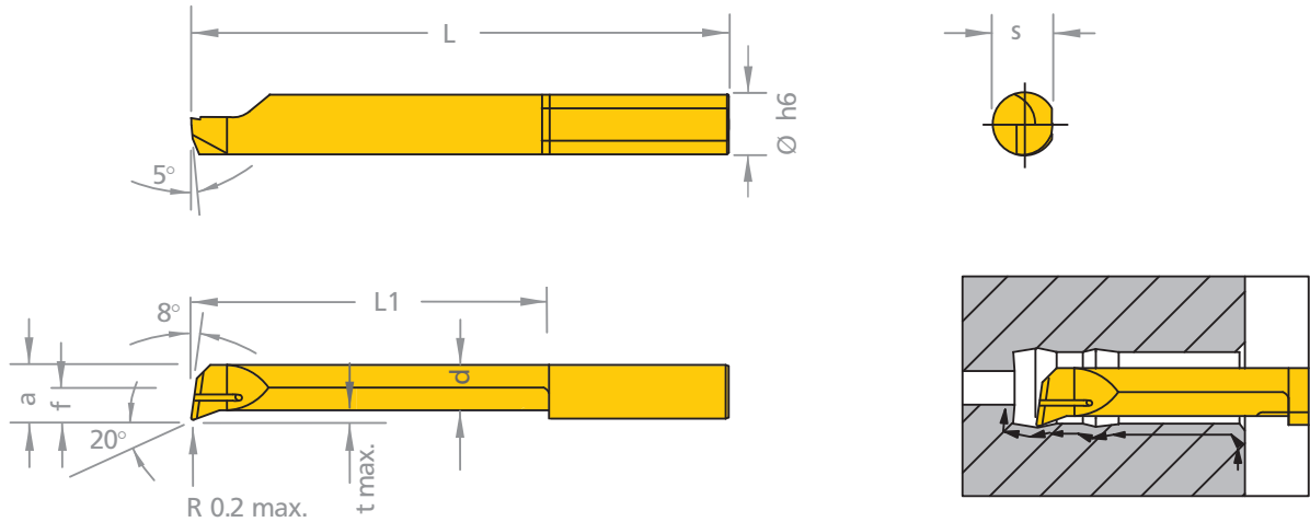
Abbildung: rechtsschneidend
